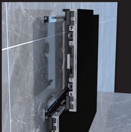
LED キャビネットを引っ掛けてねじで固定
